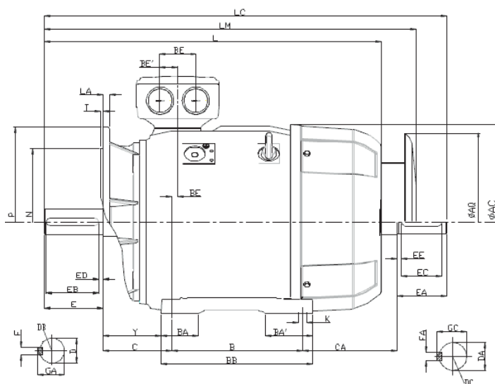
Fuß-Flanschbauformen feet / flange type of construction
